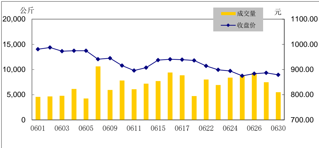
Au99.99量价图
