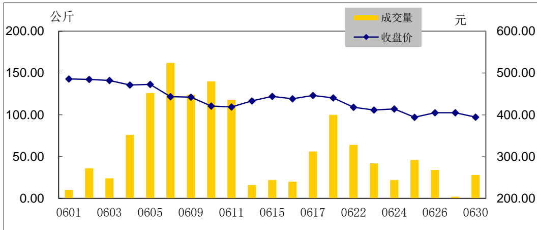
Pt99.95量价图
